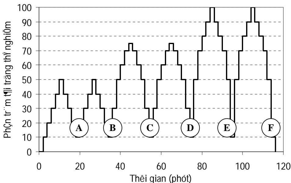
Hình B.1 - Các cấp tải và trình tự thí nghiệm lặp sáu chu kỳ
